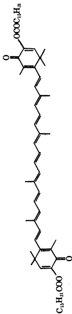
Astacein
